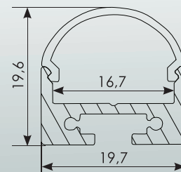
Querschnitt Aluminiumprofil (mm):
